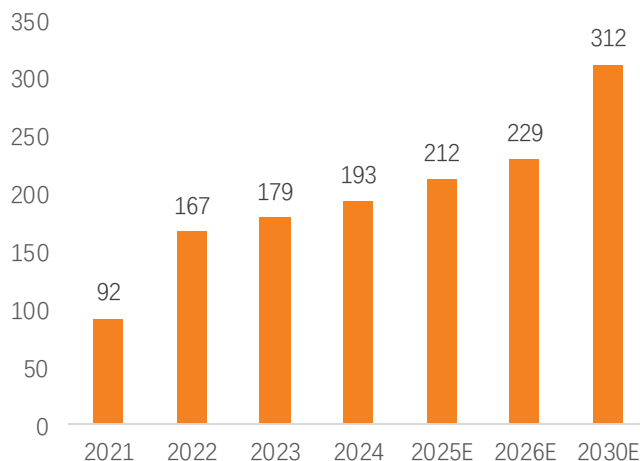
图：高效电机产量及预测（GW）
